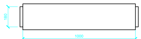
Flexibilní hlukový tlumič DN180
