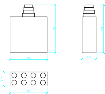
ROZDĚLOVAČ VZDUCHU CWL DN 125-180, 8 HRDEL
