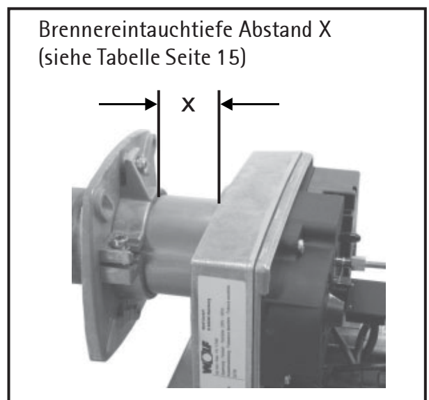
Bild: Brennereintauchtiefe
