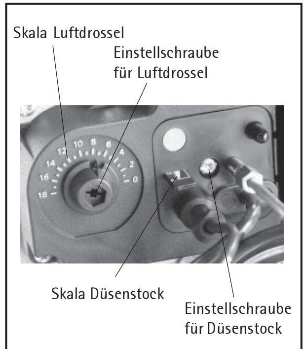
Bild: Luftregulierung
