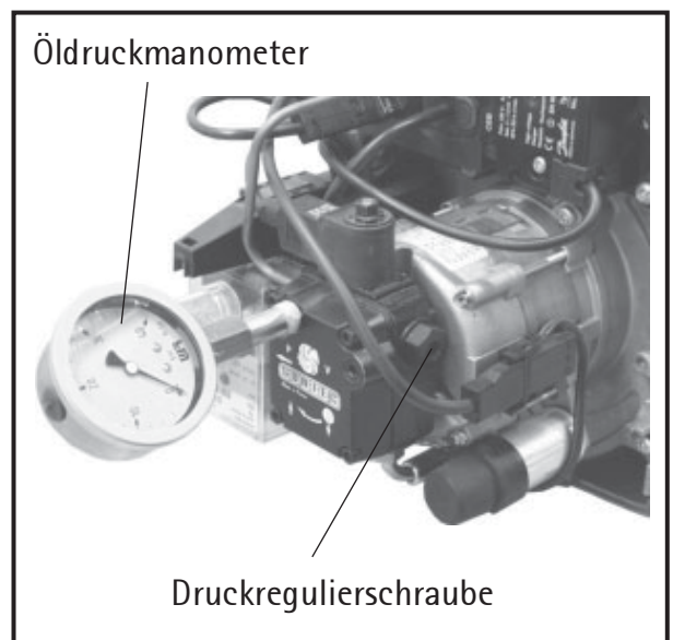
Bild: Öldruckmanometer
