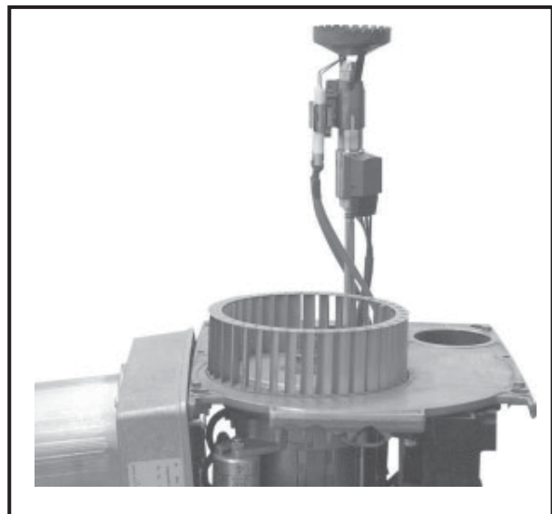
Bild: Serviceposition
