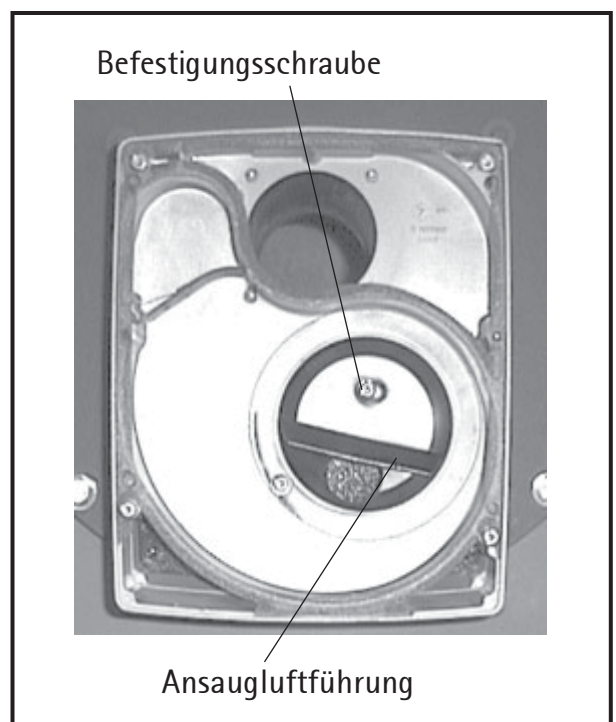
Bild: Ansaugluftführung
