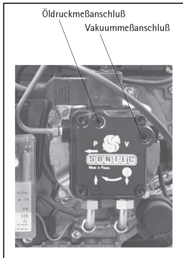
Bild: Unterdruckkontrolle
