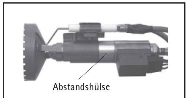
Bild: Montage Stauscheibe EK01B.3/4/5L-TH/TH1
