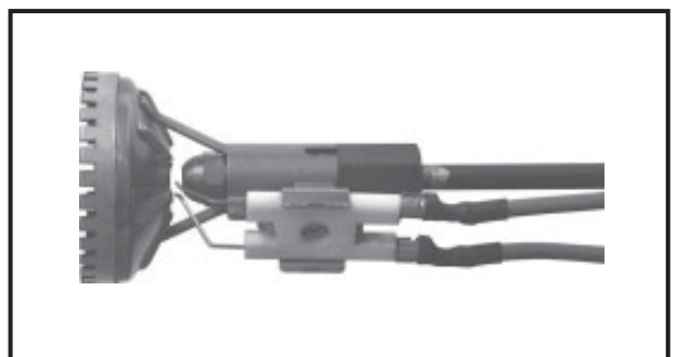
Bild: Montage Stauscheibe EK01B.7L-T
