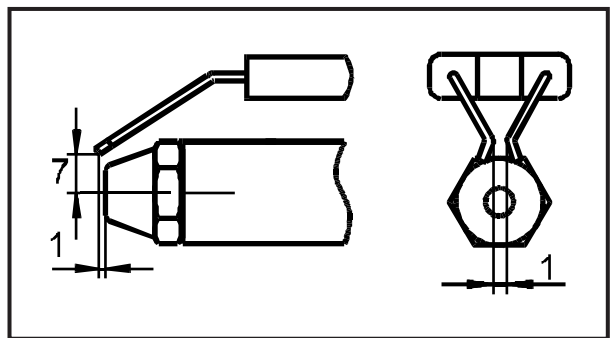
Bild: Elektrodenabstand
