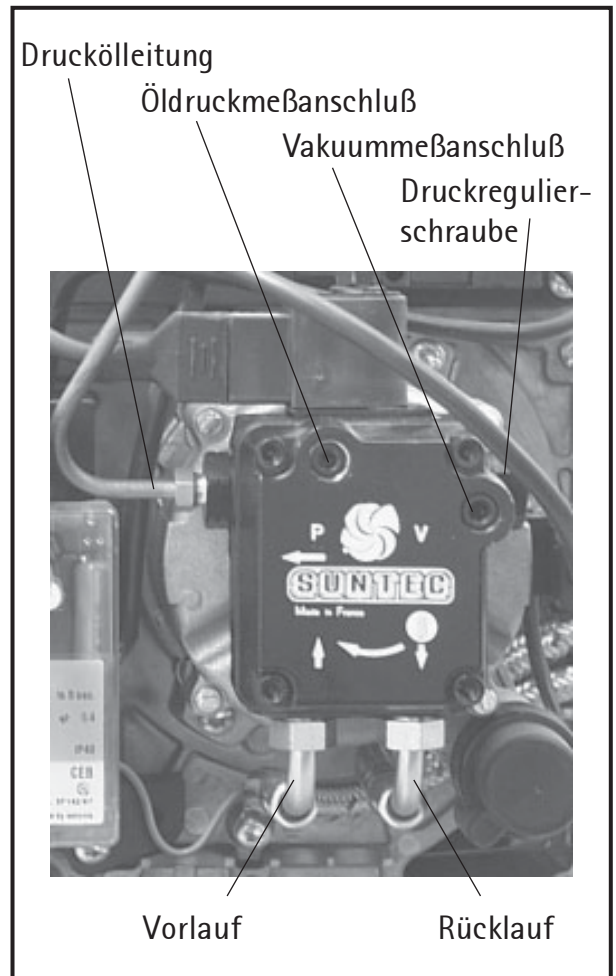
Bild: Einstellung Pumpendruck
