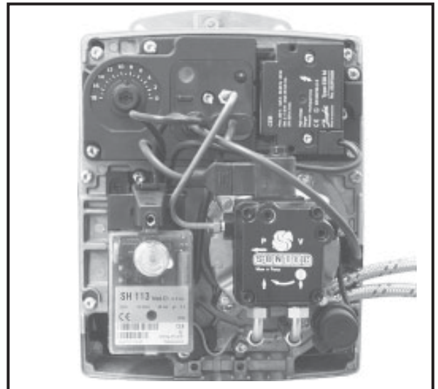
Bild: Einbaulage Brenner
