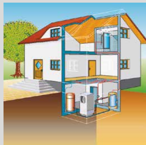
Anlagenschema - Innenaufstellung
