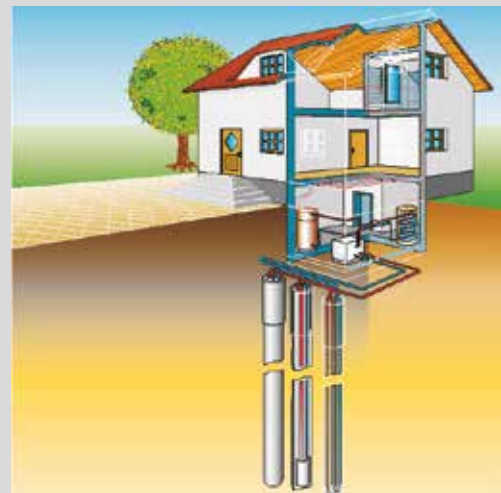
Anlagenschema - Erdsonde
