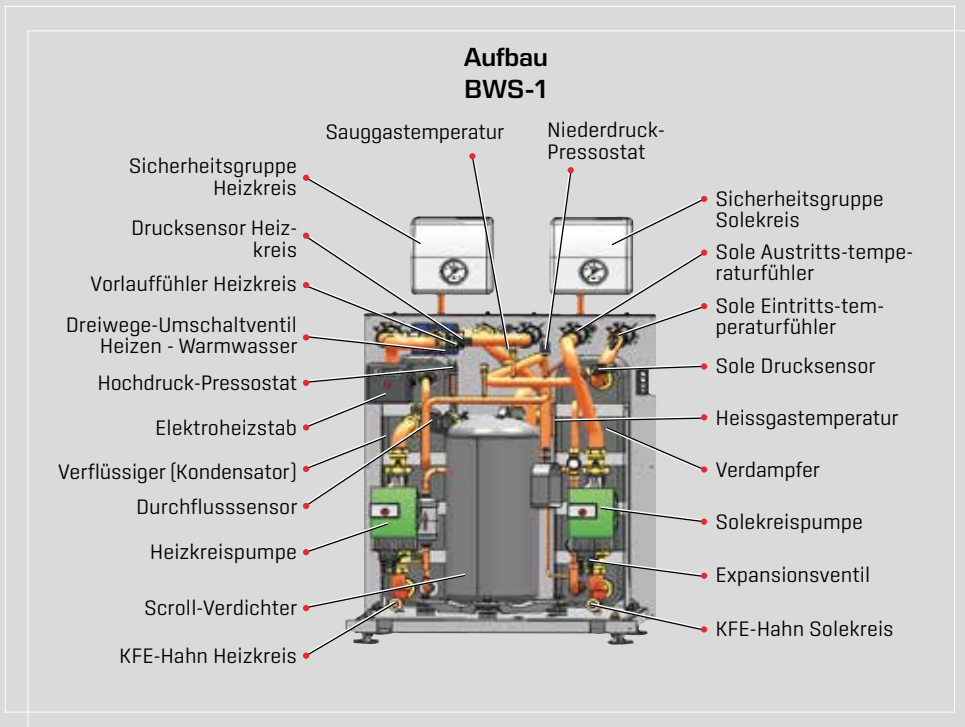
Innenaufstellung BWS-1
